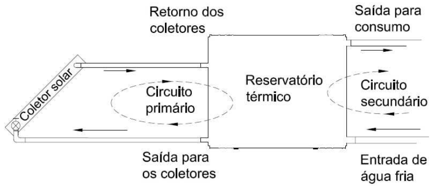
Figura 7 — A1- Esquema do SAS
