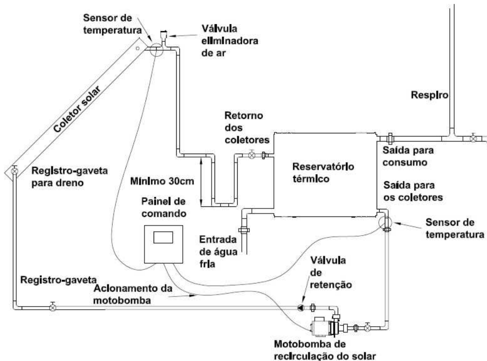
Figura 2 — Esquema de circuito para circulação forçada
