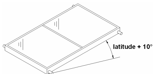
Figura 4 — Ângulo de inclinação dos coletores
