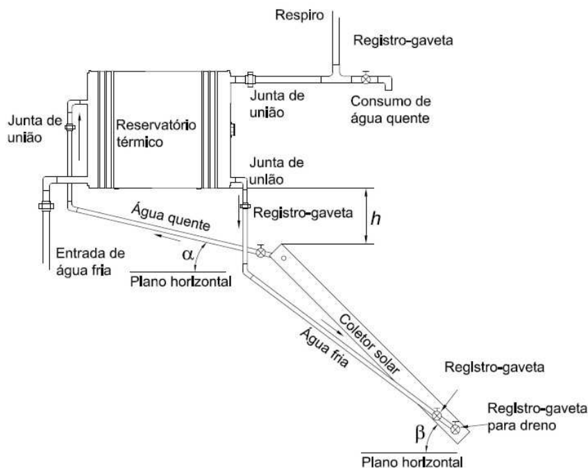
Figura 1 — Esquema de circuito para termossifão
