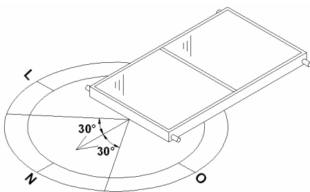
Figura 3 — Orientação geográfica dos coletores
