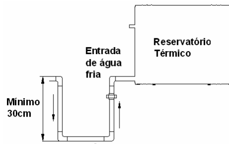
Figura 6 — Exemplo de sifão 2
