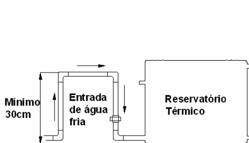
Figura 5 — Exemplo de sifão 1
